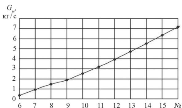
Рис. 5. Залежність витрати води на охолодження від номера компресорного ступеня, у який вона подається (другий етап досліджень)
