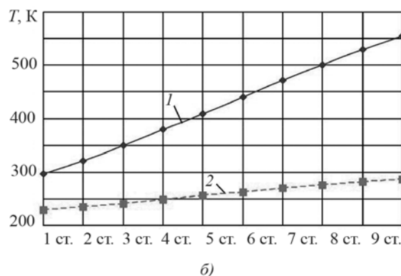
Рис. 1. Зміна температури повітря (1) і температури кипіння води при даному тиску (2) по ступенях компресорів низького (а) і високого (б) тисків
