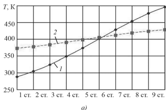
Рис. 1. Зміна температури повітря (1) і температури кипіння води при даному тиску (2) по ступенях компресорів низького (а) і високого (б) тисків
