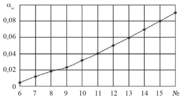
Рис. 4. Залежність відносної витрати охолоджуючої води від номера компресорного ступеня, у який вона подається (другий етап досліджень)
