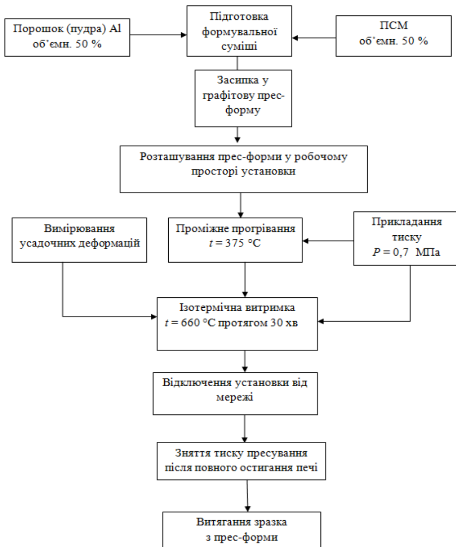
Рисунок 2 – Технологічна схема отримання зразків
