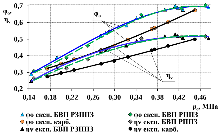
Рис. 6. Експериментальні значення коефіцієнта наповнення \eta_v та коефіцієнта надлишку продувочного повітря \phi_o двигуна з карбюратором, БВП з РЗППЗ та БВП та РЗППЗ
