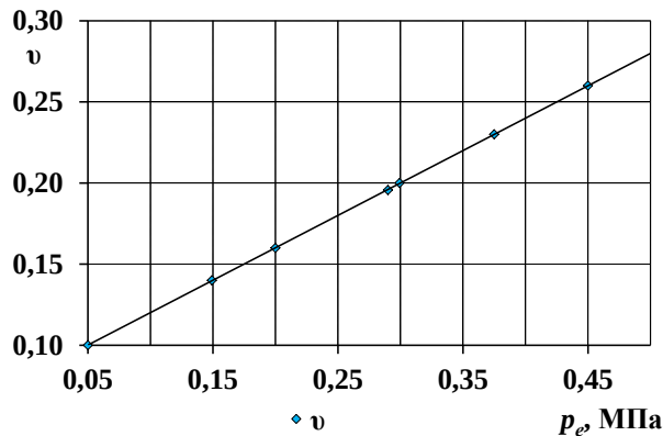
Рис. 4. Експериментальні значення коефіцієнта витоку \nu
