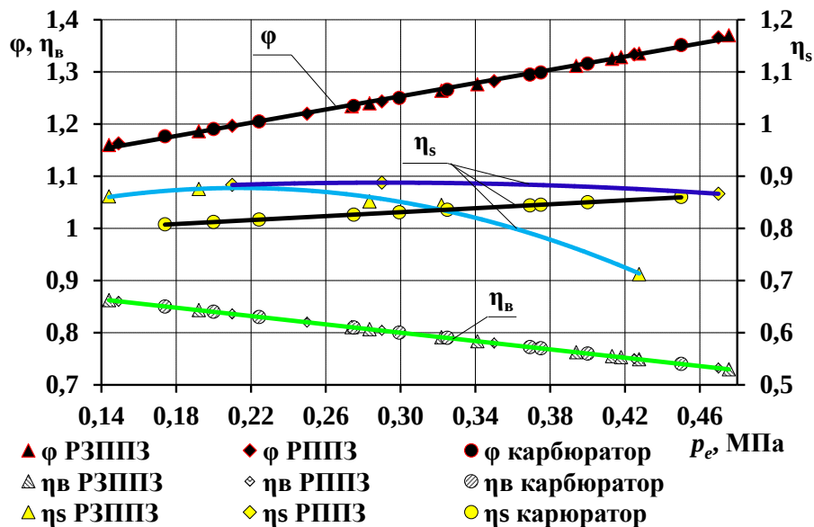
Рис. 7. Значення коефіцієнта продуктивності \phi , коефіцієнта використання продувочного повітря \eta_v та к.к.д. продуктивності \eta_s двигуна з карбюратором, БВП з РППЗ та РЗППЗ
