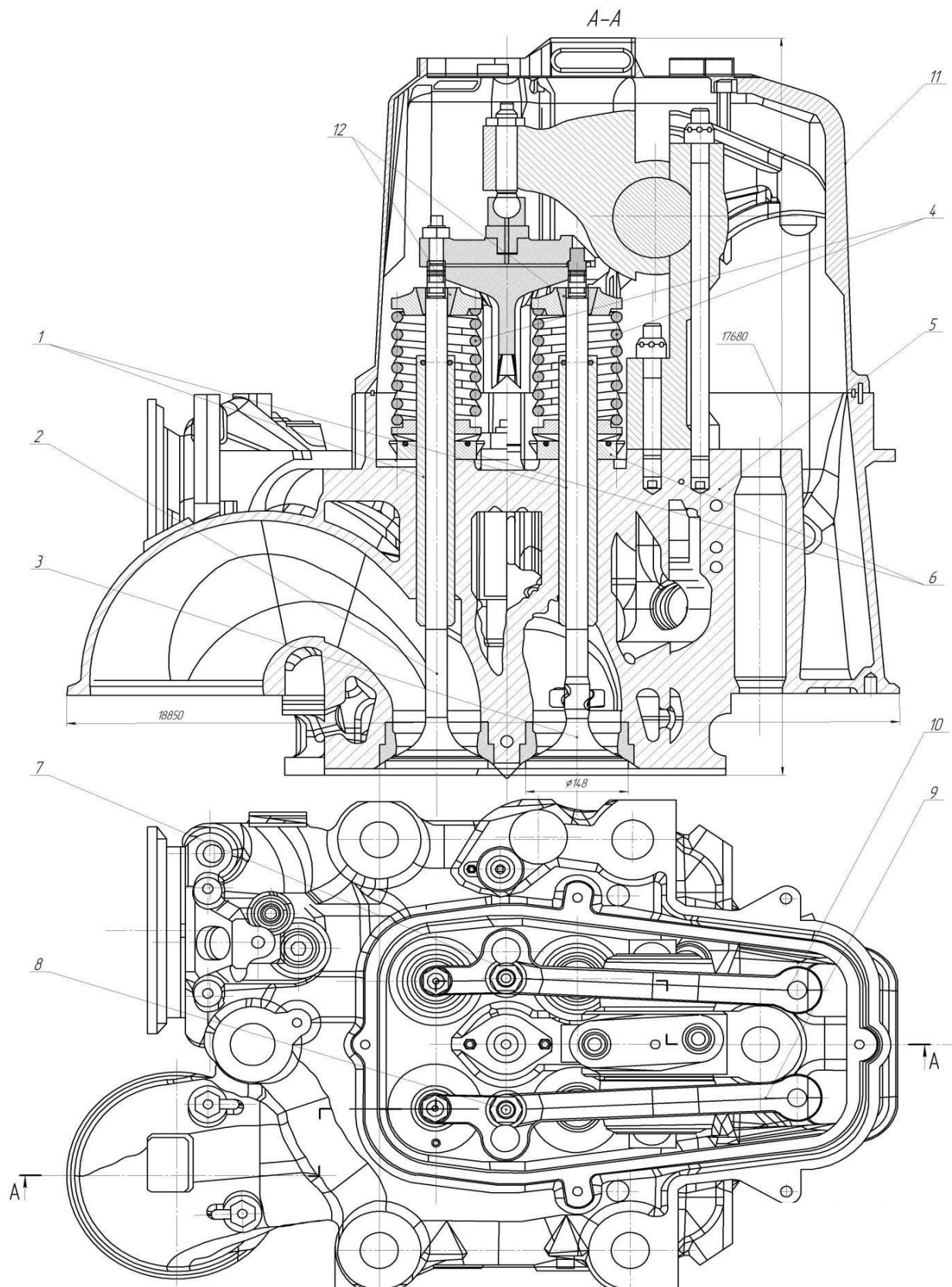
Рисунок 3.4 – Компонування деталей газорозподільного механізму у головці циліндра судноводивуна МаК 8М43С: 1 – втулка клапана; 2 – впускний клапан; 3 – випускний клапан; 4 – пружина; 5 – корпус головки циліндрів; 6 – механізм повороту клапана; 7 – комплект випускного клапана; 8 – комплект впускного клапана; 9 – рокер впускного клапана; 10 – рокер випускного клапана; 11 – кришка головки циліндра; 12 – затискний конус
