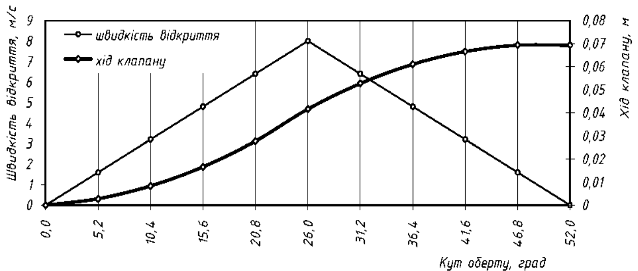
Рисунок 3.7 - Графічна схема відкриття клапанів двигуна
