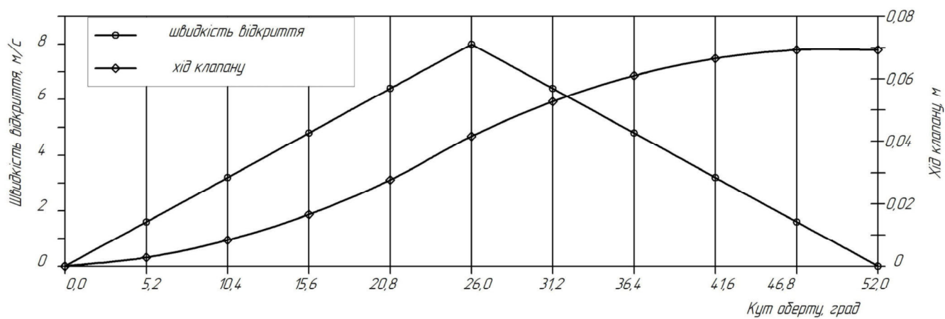
Графічна схема відкриття клапанів
