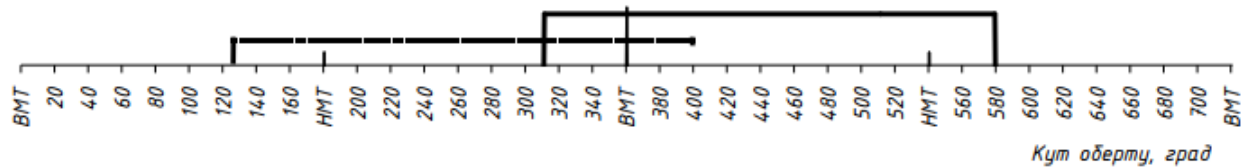
Рисунок 3.6 - Графічна схема відкриття клапанів: ----- впускний клапан; _____ пусковий клапан
