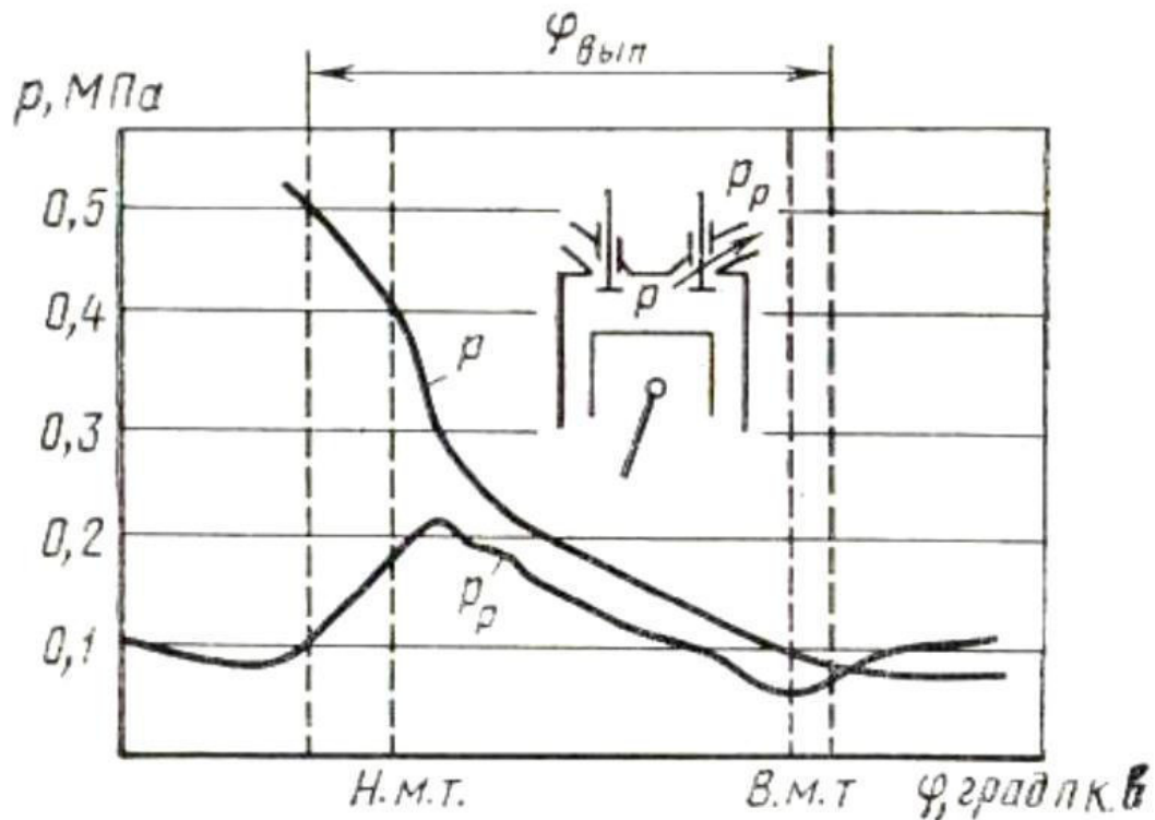
Рисунок 1.2 - Зміна тиску P_c і P_p в процесі випуску в 4 тактном ПДВЗ ( \varphi_{\text{вип}} - фаза випуску) [1 - 15]
