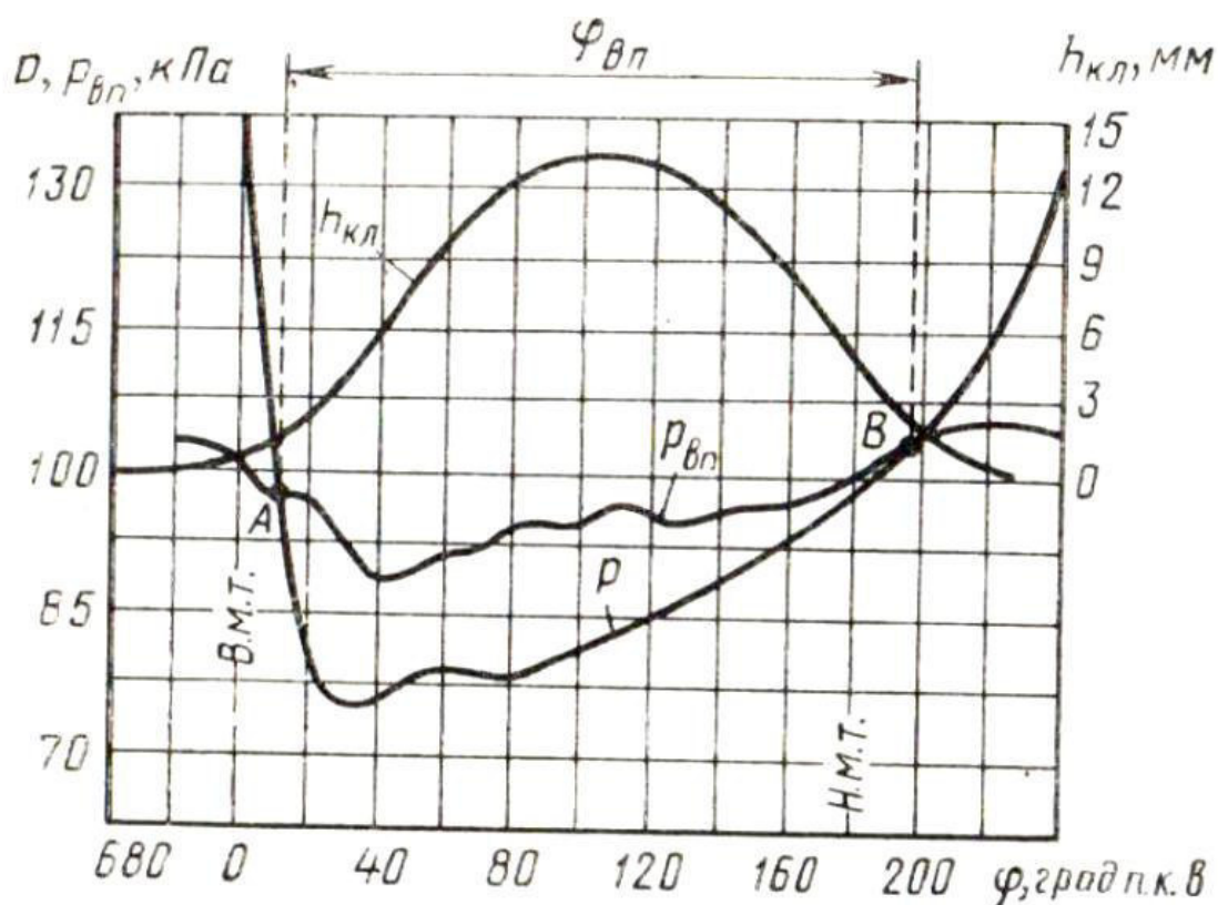
Рисунок 1.3 - Зміна тиску P_{\text{ц}} і P_{\text{вп}} в процесі випуску в 4 тактном ПДВЗ (ФВП - фаза випуску) [1 - 15]
