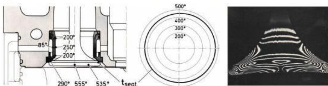
Рисунок 3.2 - Температурні поля клапана (ліворуч) та сідла (центр) та розподіл напруг в тарілці клапана (праворуч)
