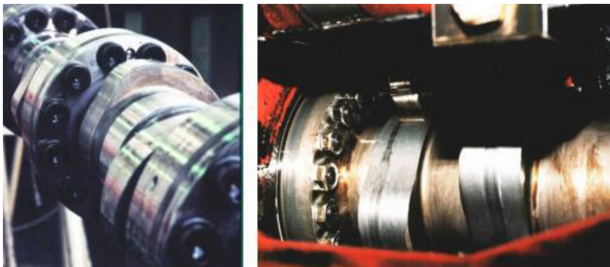
Рисунок 3.1 - Кулачки розподільного вала та клапанів дизельного двигуна МАК М32 після 15000 годин роботи
