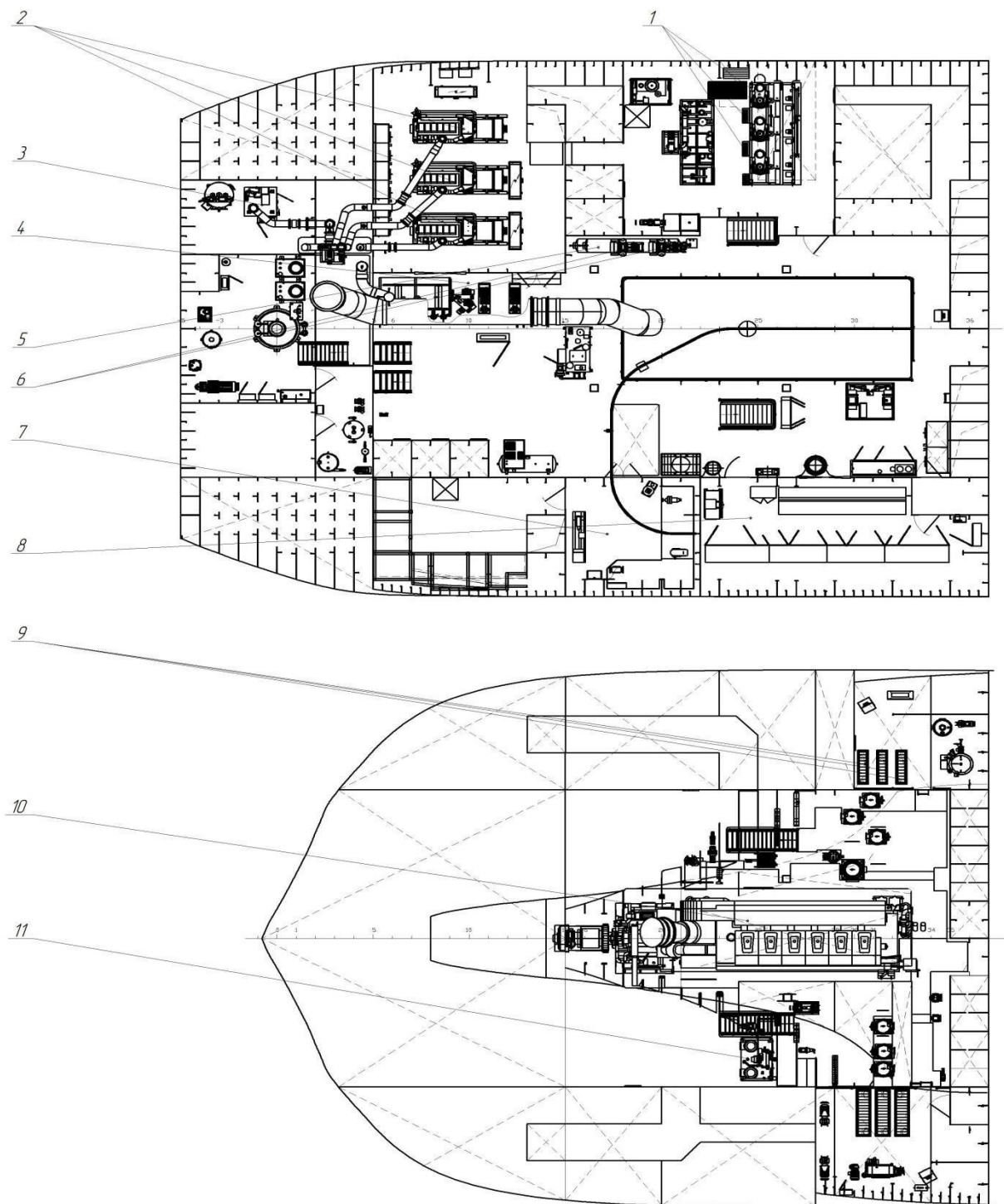
Рисунок 2.3 - Загальне розташування механізмів у машинно-котельному відділенні судна: 1 – масляні сепаратори; 2 – дизель-генератори; 3 – інсенератор; 4 – ділянка підготовки палива; 5 – повітряні ресивери; 6 – повітряні компресори; 7 – суднова майстерня; 8 – центральний пост керування; 9 – масляні охолоджувачі; 10 – головний двигун; 11 – ділянка ремонту паливної апаратури
