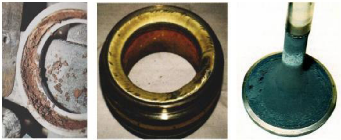
Рисунок 3.3 - Пошкодження сідел клапанів (зліва та посередині) та випускний клапан дизеля Vasa 32 після 10000 годин роботи на важкому паливі (справа)
