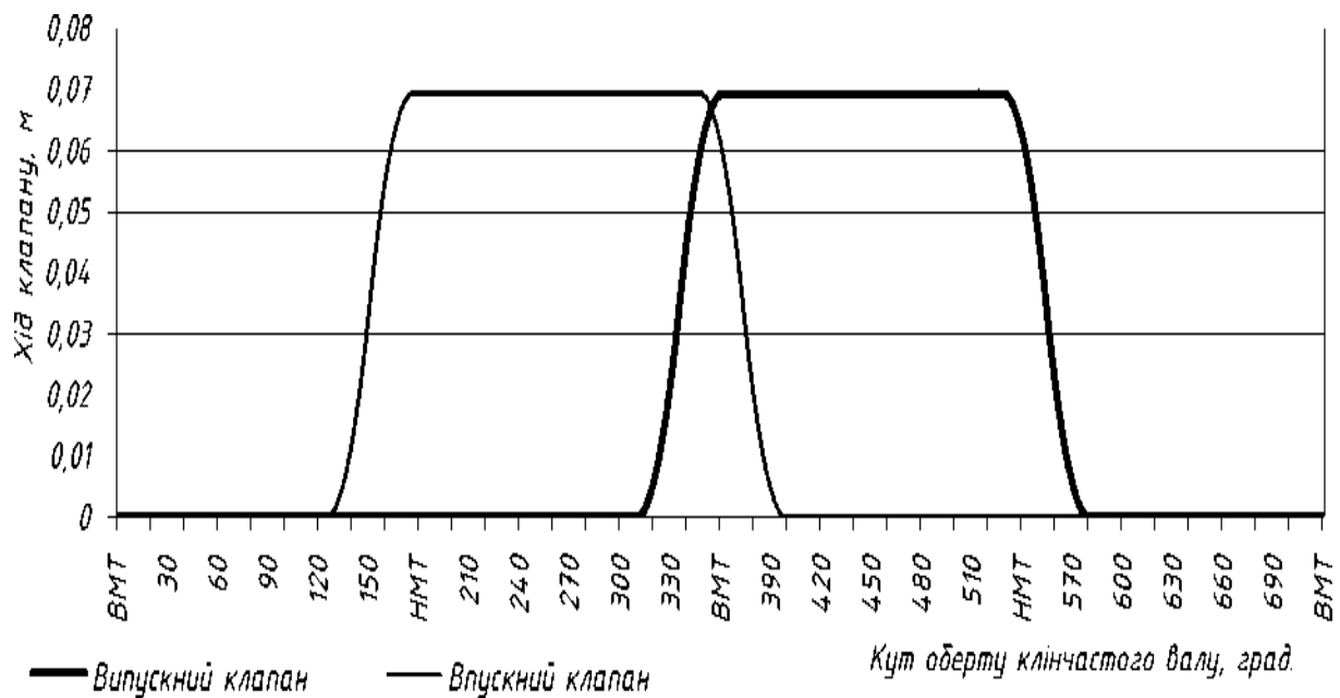
Рисунок 3.8 - Діаграма відкриття клапанів двигуна
