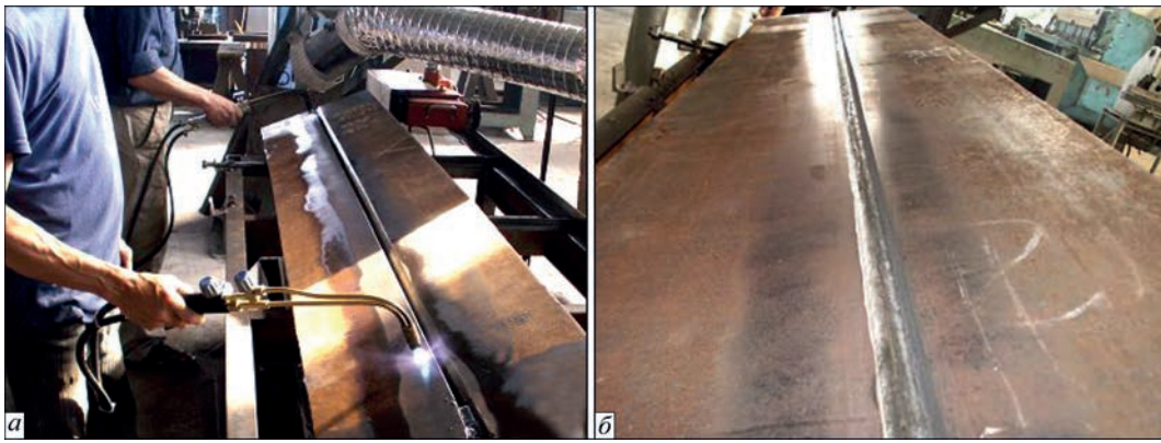
Рис. 1. Зовнішній вигляд контрольних зварних з'єднань до (а) та після (б) зварювання
