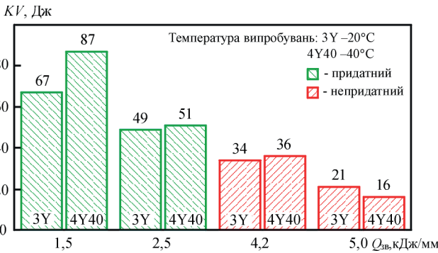
Рис. 3. Залежність середньої роботи удару металу шва ( KV ) від погонної енергії зварювання ( Q_{зв} ); температура випробувань: 3Y -20 °С; 4Y40 -40 °С
