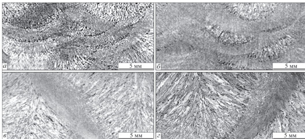
Рис. 4. Макроструктура наплавленого металу (рис. 2, зона А): а – Q_{\text{зв}} = 1,5 кДж/мм; б – 2,5; в – 4,2; з – 5,0
