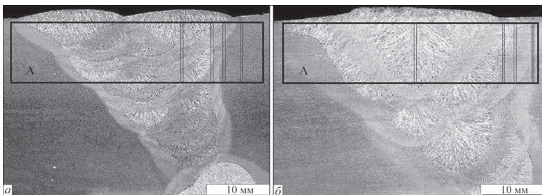
Рис. 2. Макроструктура зварних з'єднань сталі E36: а – Q_{36} = 1,5 кДж/мм; б – 5,0
