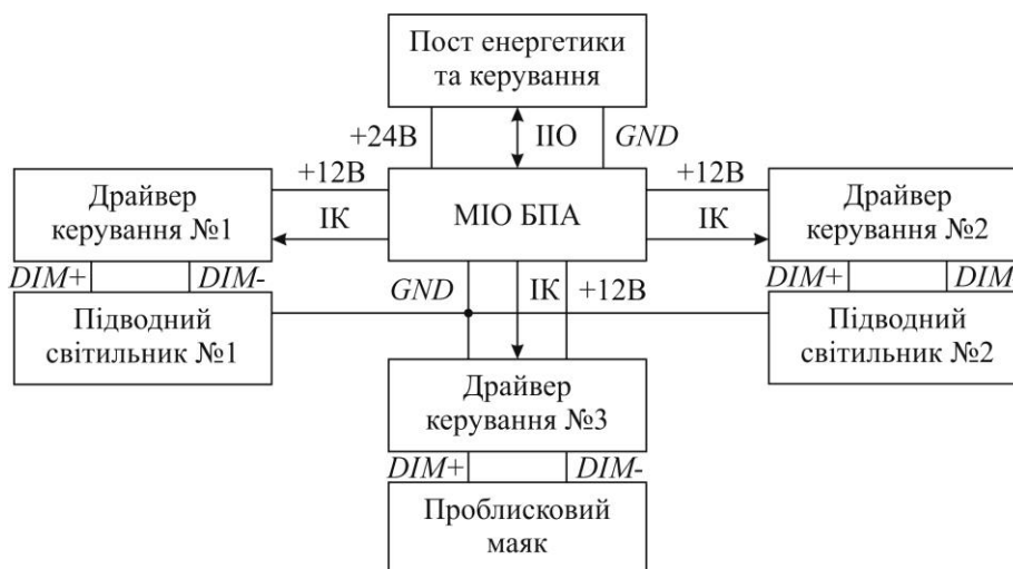
Рисунок 1 – Структурна схема системи освітлення БПА
