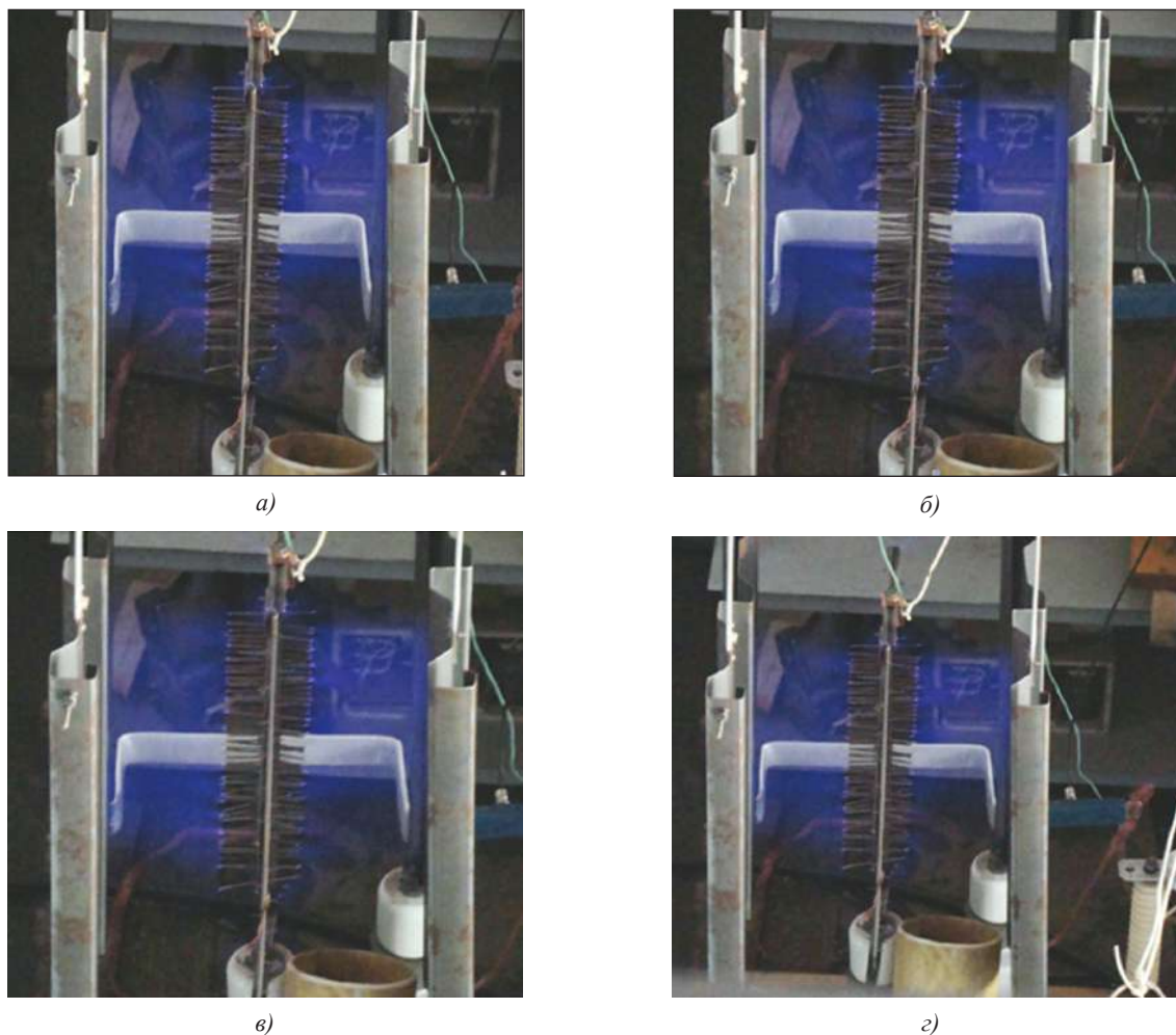
Рис. 5. Объемный разряд при различных скоростях потока воздуха v_n : а) v_n = 0 м/с; б) v_n = 10 м/с; в) v_n = 15 м/с; з) v_n = 20 м/с
