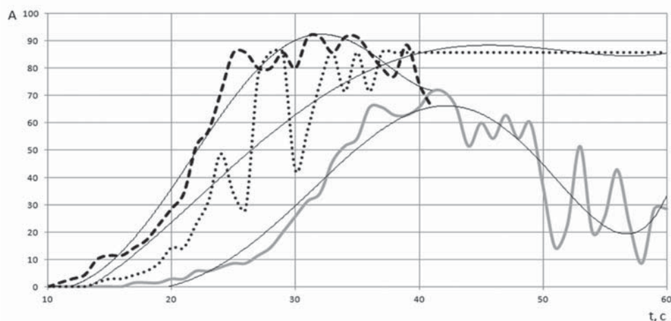
Рис. 7. Коливання ніхромового електрода-струни ( d = 0,35 мм): — 19,39 кВ; ..... — 20,78 кВ; — · — 22,16 кВ
