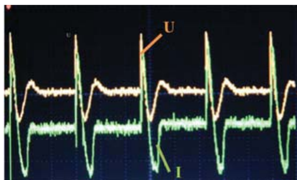
Рис. 2. Осциллограмма тока и напряжения высокочастотного стримерного разряда (развертка 250 мкс/дел.)
