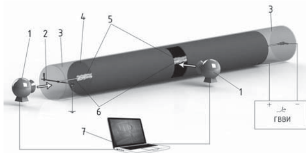
Рис. 1. Экспериментальный стенд с коаксиальной цилиндрической электродной системой:
