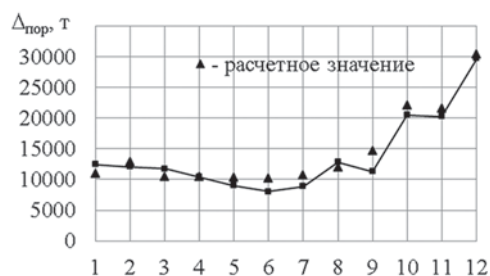
Рис. 1. Расчет водоизмещения порожнем буровых судов
