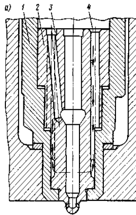
Рис. 3.10 – Розпилювач з охолодженням.
