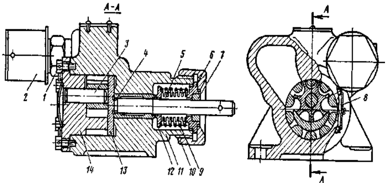
Рис. 3.8 – Паливний насос:
