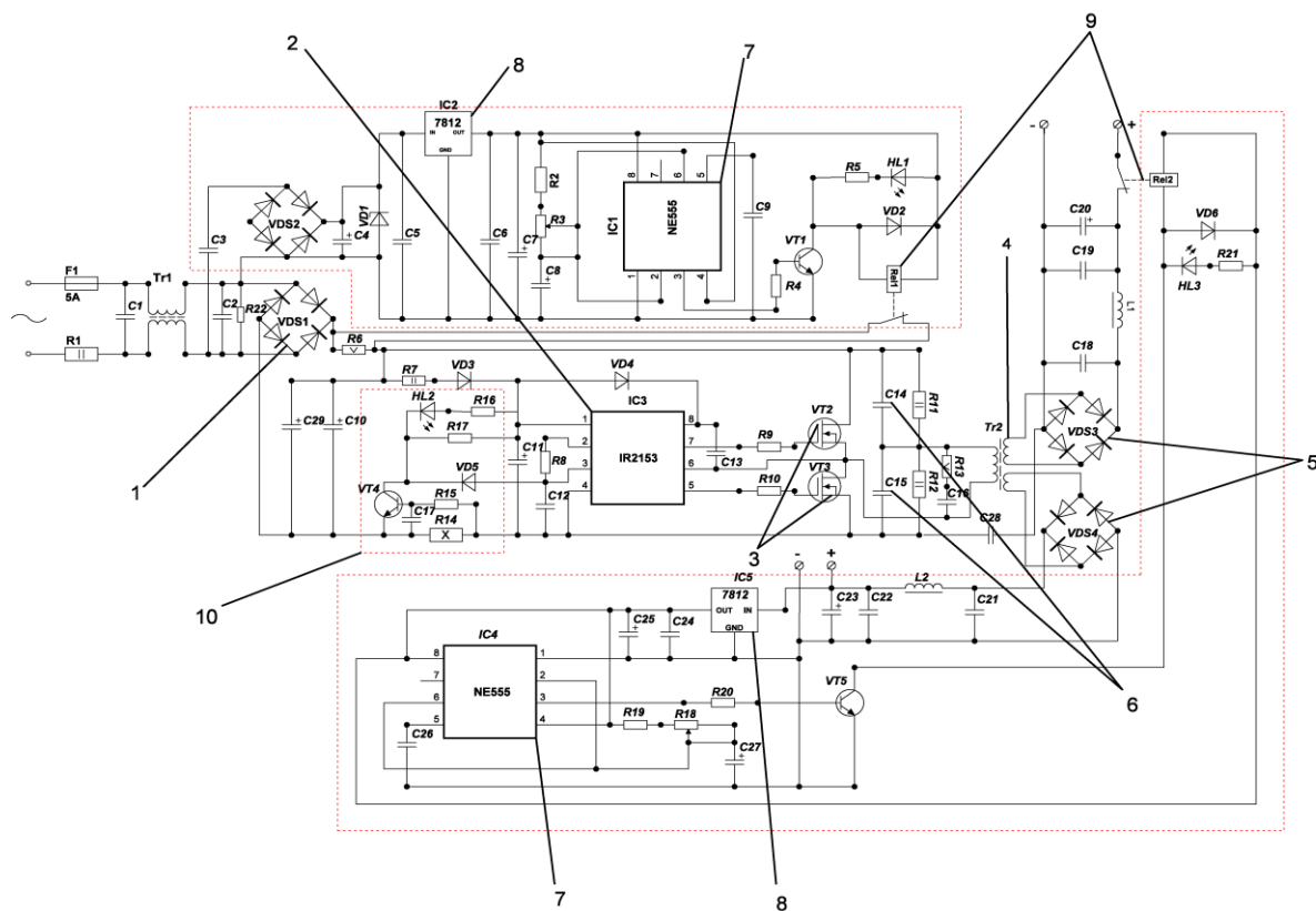
Рис. 1 - Вдосконалена схема блока живлення лабораторного стенда
