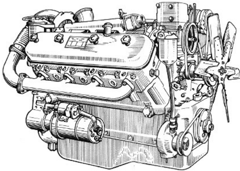
Рисунок 1.1 Двигун ЯМЗ-238
