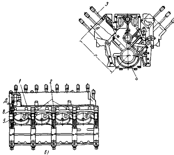
Рисунок 1.3 Блок-картер двигуна ЯМЗ-238
