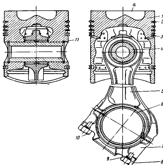
Рисунок 1.5 Шатунно-поршнева група двигуна ЯМЗ-238
