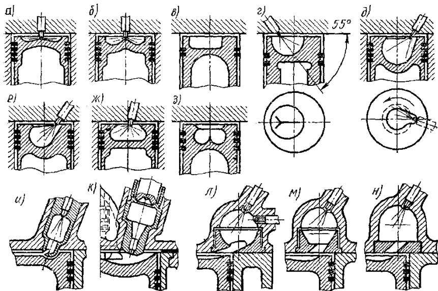
Рисунок 3.1 Форми камер згорання автотракторних дизелів
