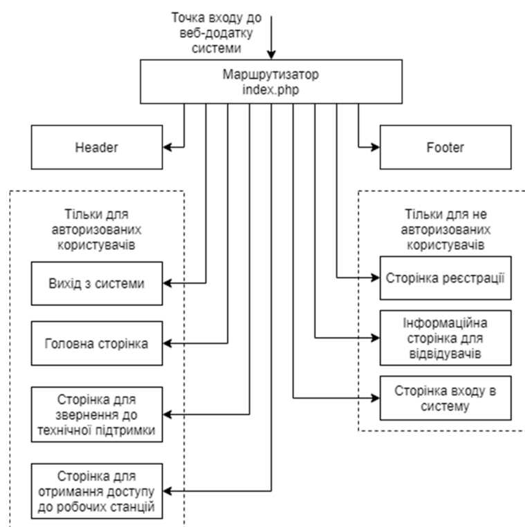
Рис. 1. Структурна схема веб-додатку
