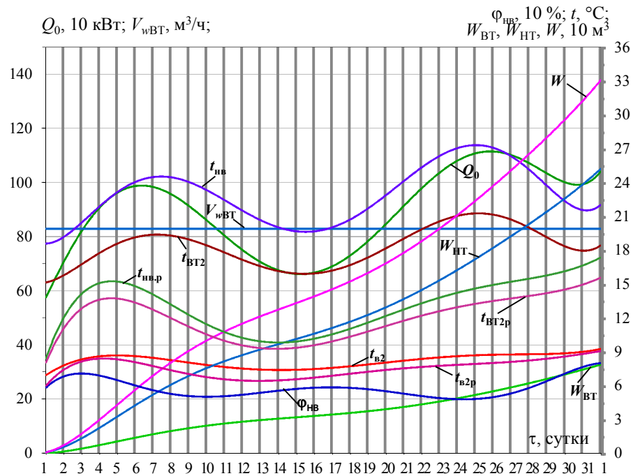
Рис. 3. Текущие значения температуры t_{нв} и относительной влажности \phi_{нв} наружного воздуха, температуры воздуха t_{БТ2} на выходе из ВО_{БТ} и t_{в2} на выходе из ВО_{НТ} , соответствующих значений температуры точки росы t_{нв,р} , t_{БТ2,р} и t_{в2,р} , а также тепловой нагрузки Q_0 на весь ВО, часового расхода охлаждающей воды G_w в ВО_{БТ} , часовых суммарных расходов конденсата V , выпадающего в ВО_{БТ} и ВО_{НТ} , соответствующее количество конденсата W , образующегося в двухступенчатом ВО, W_{БТ} – в ВО_{БТ} , W_{НТ} – в ВО_{НТ} (расход воздуха 40 кг/с, расход холодной воды 80 т/ч) в течение июля 2015 г.: проектные q_{0,БТ} = 10 кВт/(кг/с); q_{0,НТ} = 24 кВт/(кг/с); q_0 = 34 кВт/(кг/с) для климатических условий г. Южноукраинск, Николаевская обл.
