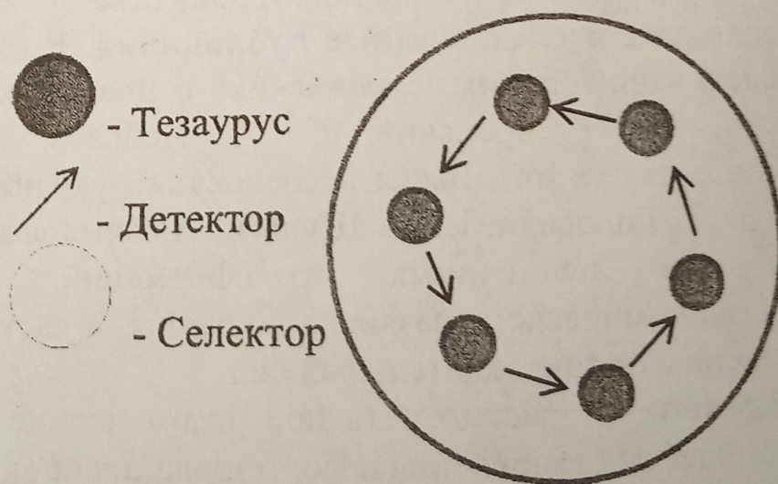
Рис. 1. Схема действия социальной системы
