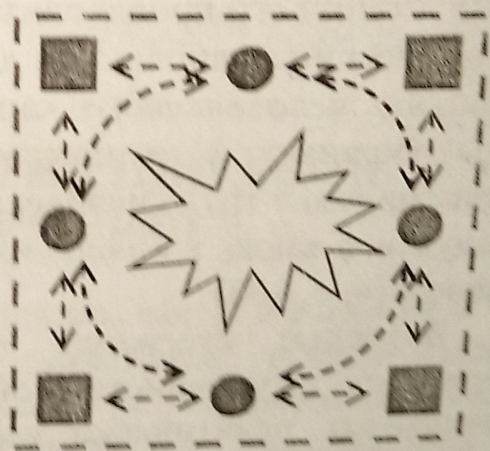
Рис. 2. Схема селекторного коллапса социальной системы
