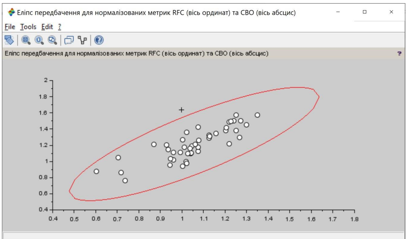
Рисунок 3.8. – Вихід точки з координатами, які відповідають значенням нормалізованих метрик RFC та CBO застосунку Metro_systems, за еліпс передбачення
