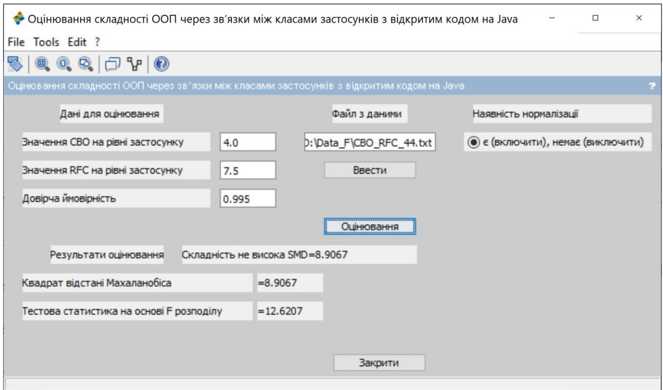
Рисунок Д.3 – Результати роботи програми після натискання на командну кнопку «Оцінювання» у разі, коли радіо кнопка включена та введені значення метрик СВО та RFC застосунку з не високою складністю ООП
