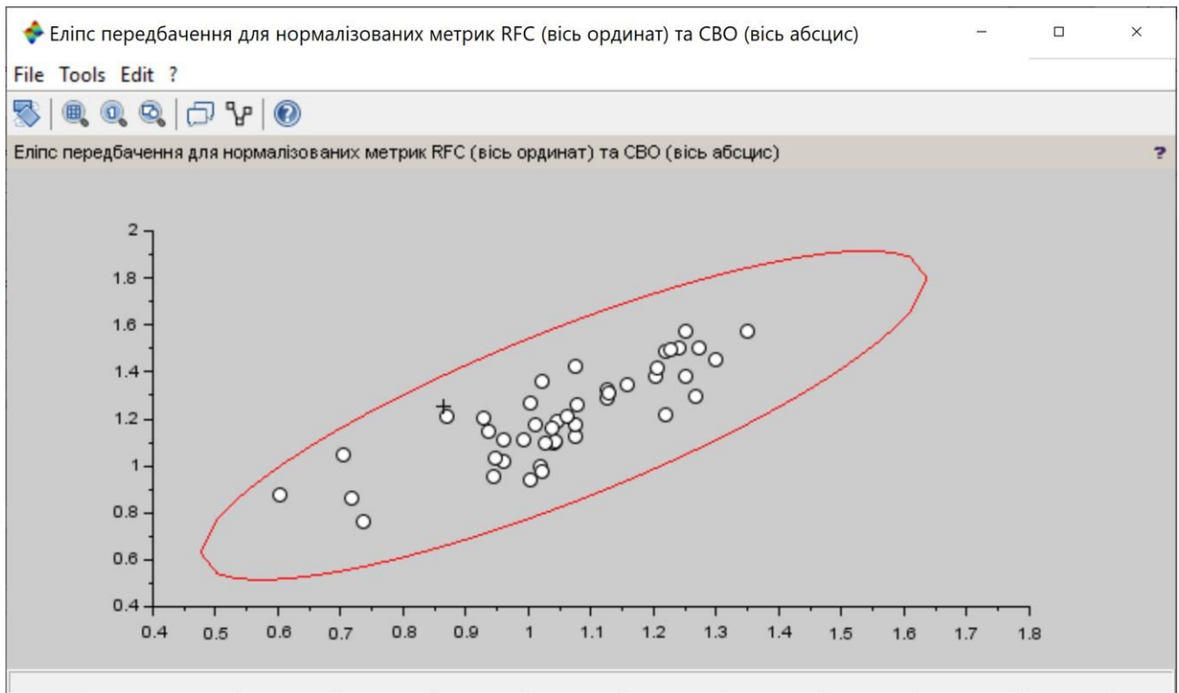
Рисунок 3.9. — Точка з координатами, які відповідають значенням нормалізованих метрик RFC та CBO застосунку TuxGuitar, що знаходиться всередині еліпсу передбачення
