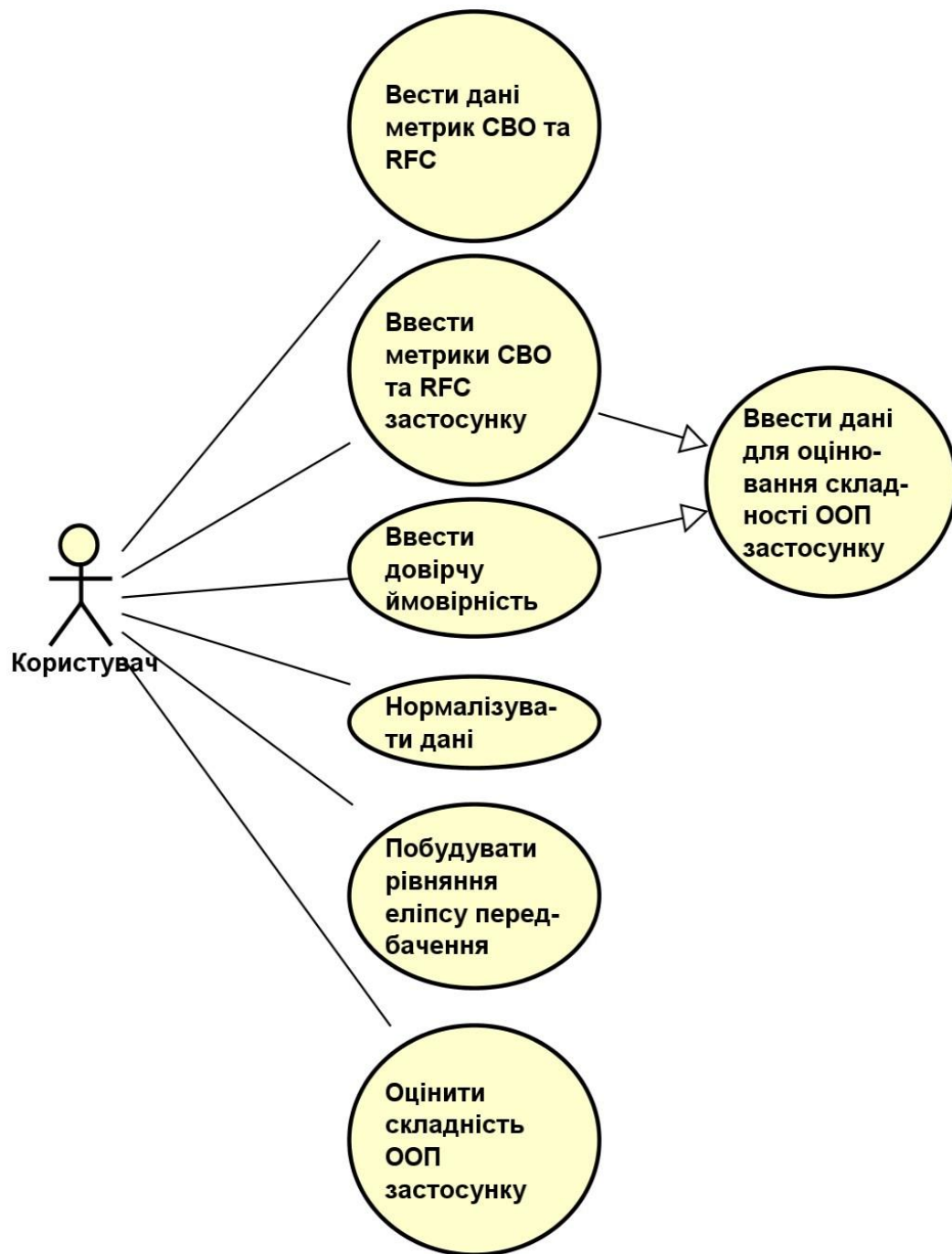
Рисунок 3.1 – Діаграма варіантів використання програми для оцінювання складності ООП через зв'язки між класами застосунків з відкритим кодом на Java
