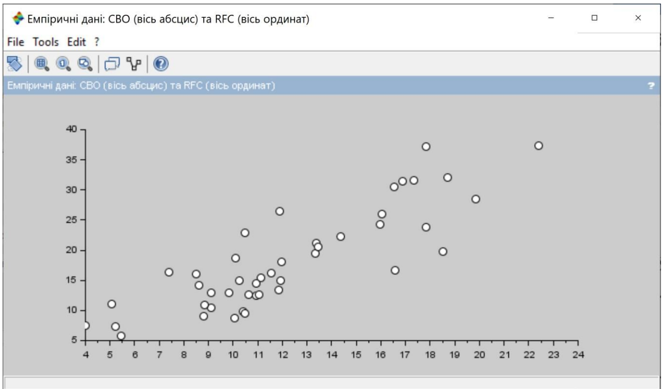
Рисунок 3.5. – Емпіричні дані з метрик CBO та RFC 44 застосунків з відкритим кодом на Java
