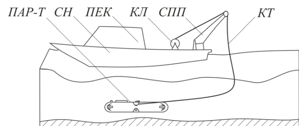
Рис. 1. Самохідна прив'язна підводна вантажна система: ПАР-Т — підводний апарат-робот; СН — судно-носіє; ПЕК — пост енергетики й керування; КЛ — кабельна лебідка; СПП — спуско-підйомний пристрій; КТ — кабель-трос
