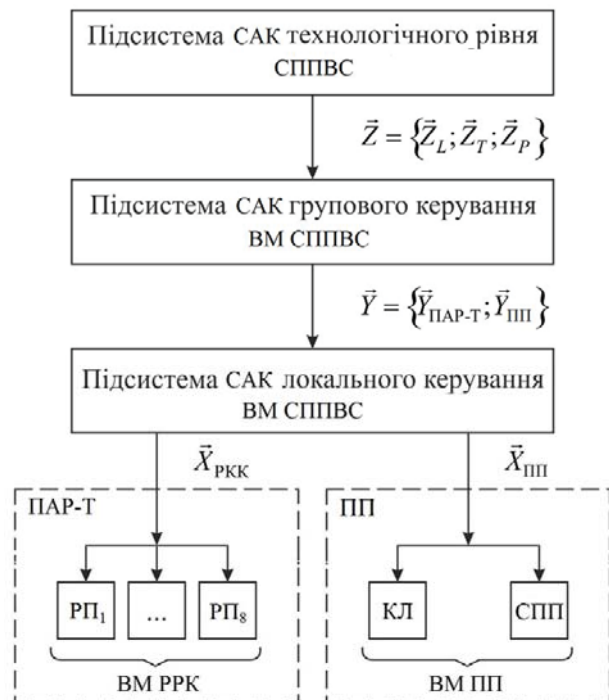
Рис. 2. Узагальнена структура системи автоматичного керування СППВС
