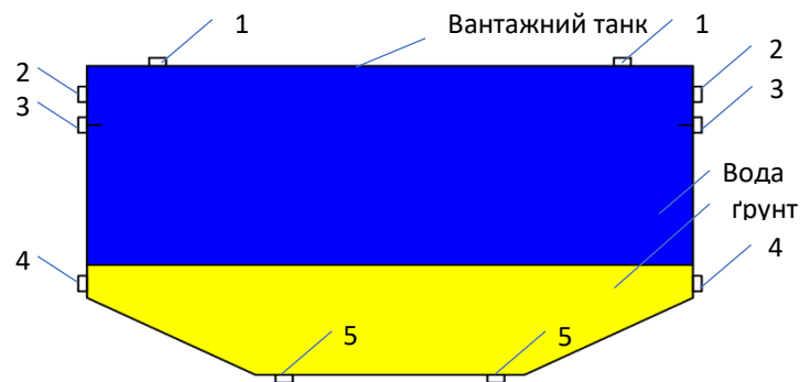
Рисунок 1 – Розташування датчиків для контролю вантажного танку
