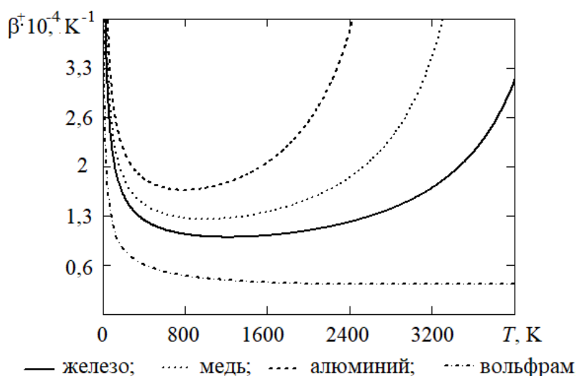
Рисунок 2 – Графік залежності коефіцієнта лінійного (теплового) розширення від температури (при розширенні металу) для деяких металів
