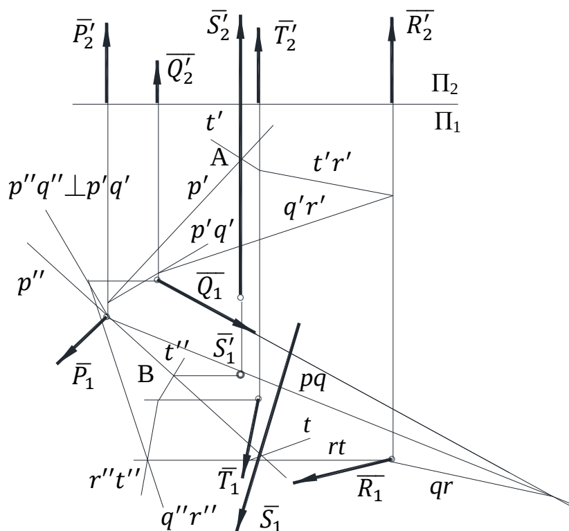
Рис.6. Побудова горизонтальної проекції \overline{S_1} рівнодіючої головного вектора
