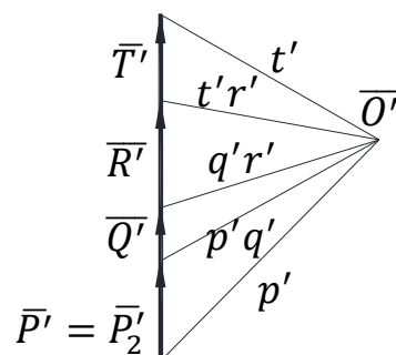
Рис. 2. План сил для вертикальних складових
