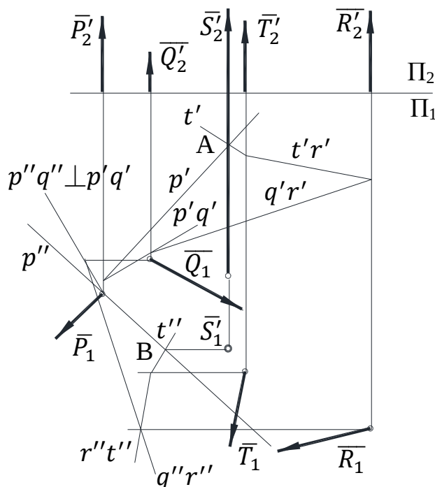
Рис. 4. Визначення горизонтальної точкової проекції \bar{S}'_1 рівнодіючої
