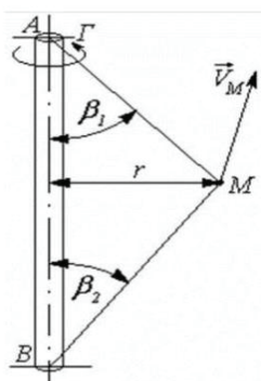
Рис. 3. Поле швидкостей потенційного вихору
