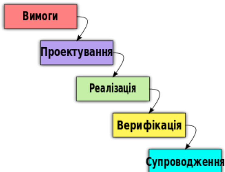
Рис. 2.1. Водоспадна модель
